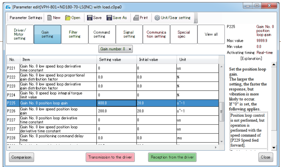
參數編輯畫面
