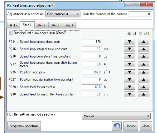
即時伺服調整畫面
