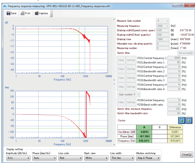
頻率響應測量畫面
