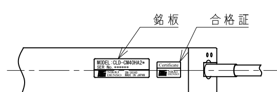
Y矢視図 (銘板貼付位置指示図)
