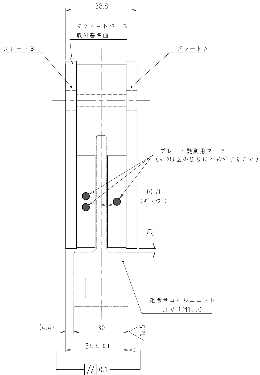
A-A'断面
